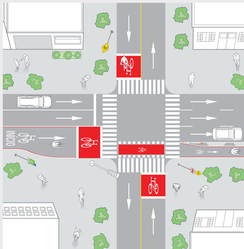
Desenho esquemático de interseção de início de ciclovia unidirecional. Fonte: ITDP Brasil (adaptação do manual “Ciclociudades: Manual integral de movilidad ciclista para ciudades mexicanas”, publicado em 2011 pelo ITDP México).
