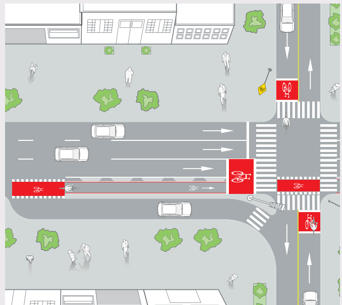
Desenho esquemático de interseção em via com conversão livre à direita e ciclovia unidirecional. Fonte: ITDP Brasil (adaptação do manual “ Ciclociudades: Manual integral de movilidad ciclista para ciudades mexicanas ”, publicado em 2011 pelo ITDP México).
