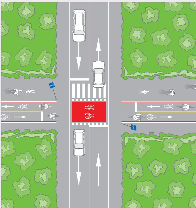
Desenho esquemático de interseção não semaforizada em ciclovia bidirecional de traçado independente e rodovia. Fonte: ITDP Brasil (adaptação do manual “Ciclociudades: Manual integral de movilidad ciclista para ciudades mexicanas”, publicado em 2011 pelo ITDP México).
