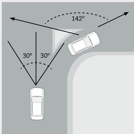
Ângulo inadequado para conversão à direita. Fonte: ITDP Brasil (adaptação de FHWA, 2004 e do manual “Ciclociudades: Manual integral de movilidad ciclista para ciudades mexicanas”, publicado em 2011 pelo ITDP México).
