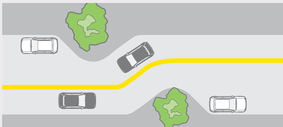
Desenho ilustrativo de chicana associada à estacionamentos em bordos opostos. Fonte: ITDP Brasil (adaptação do manual “ Ciclociudades: Manual integral de movilidad ciclista para ciudades mexicanas ”, publicado em 2011 pelo ITDP México).
