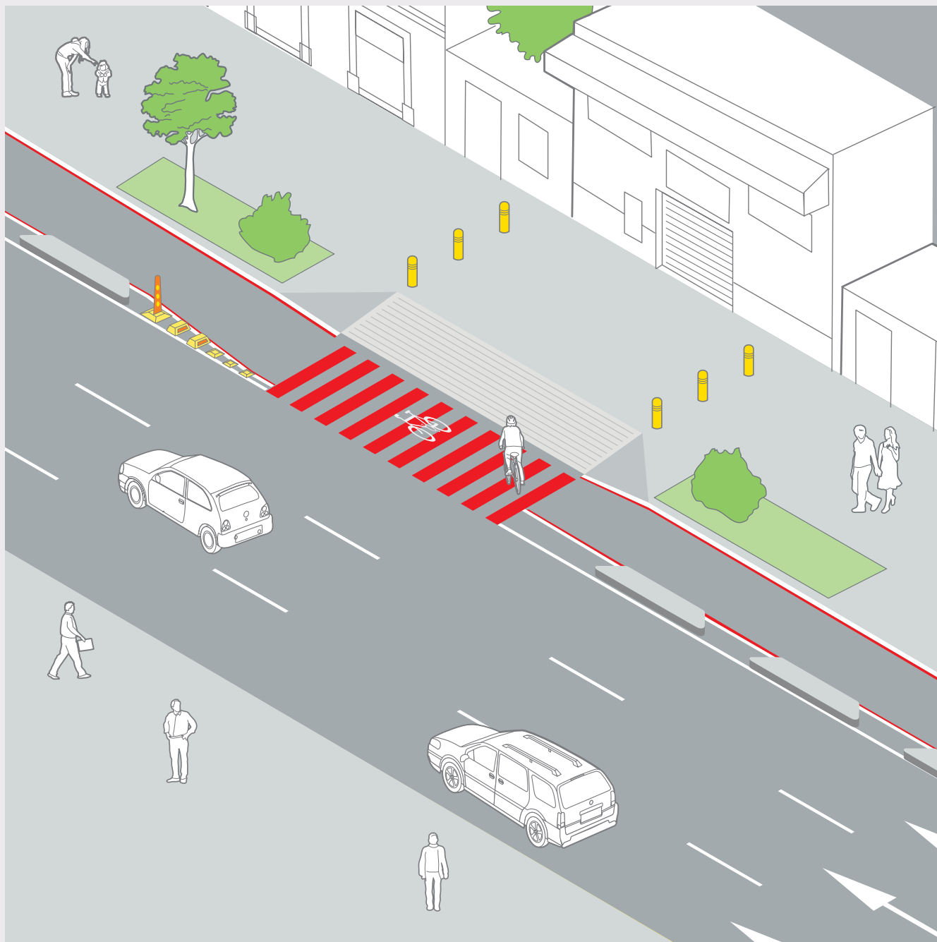
Desenho esquemático do tratamento de acessos veiculares. Fonte: ITDP Brasil (adaptação do manual “ Ciclociudades: Manual integral de movilidad ciclista para ciudades mexicanas ”, publicado em 2011 pelo ITDP México).
