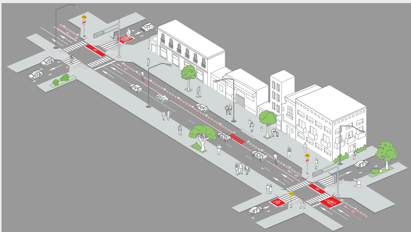
Desenho esquemático de caráter ilustrativo de uma ciclovia unidirecional em uma via com três faixas de rolamento em sentido único para o tráfego de veículos motorizados. Fonte: ITDP Brasil (adaptação do manual " Ciclociudades: Manual integral de movilidad ciclista para ciudades mexicanas ", publicado em 2011 pelo ITDP México).
