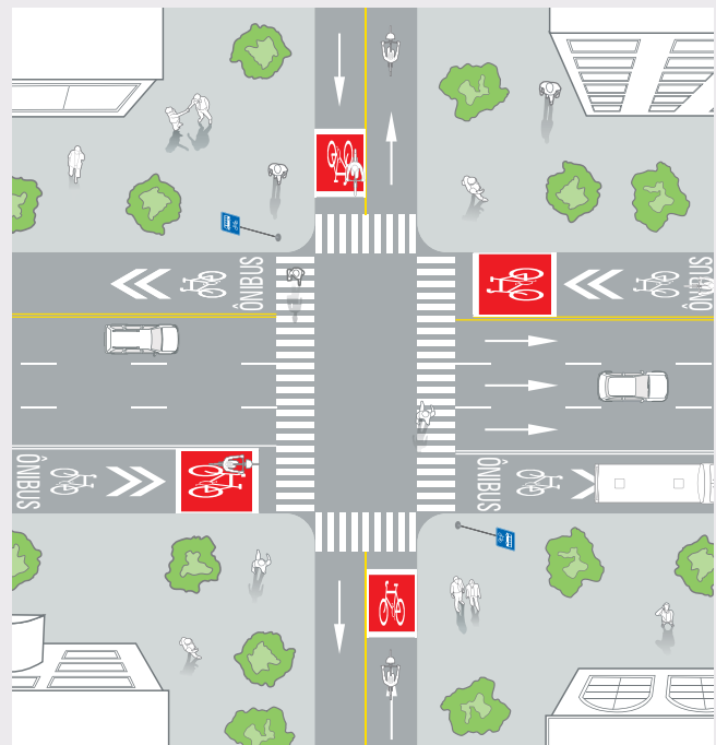
Desenho esquemático de interseção em via compartilhada entre transporte público e bicicleta. Fonte: ITDP Brasil (adaptação do manual “Ciclociudades: Manual integral de movilidad ciclista para ciudades mexicanas”, publicado em 2011 pelo ITDP México).
