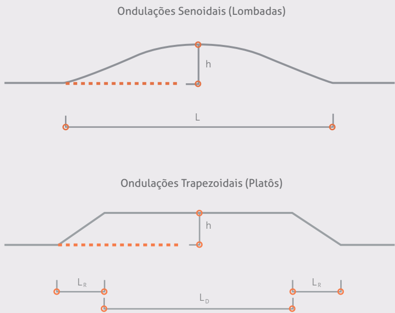
Dimensões recomendadas para ondulações transversais a pista, na Dinamarca
