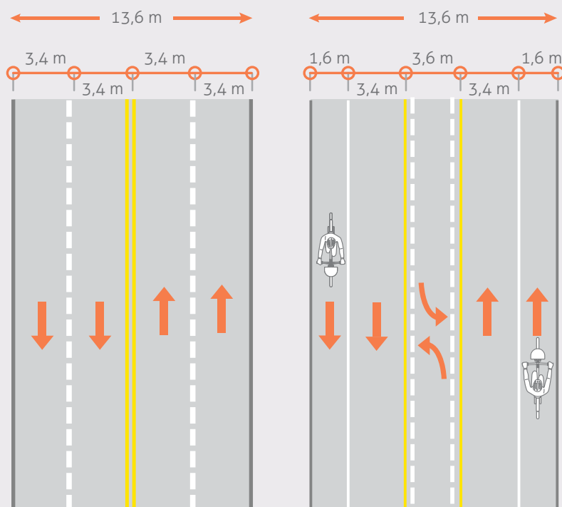
Desenho esquemático da “dieta da via”. Fonte: ITDP Brasil (adaptação do manual “Ciclociudades: Manual integral de movilidad ciclista para ciudades mexicanas”, publicado em 2011 pelo ITDP México).
