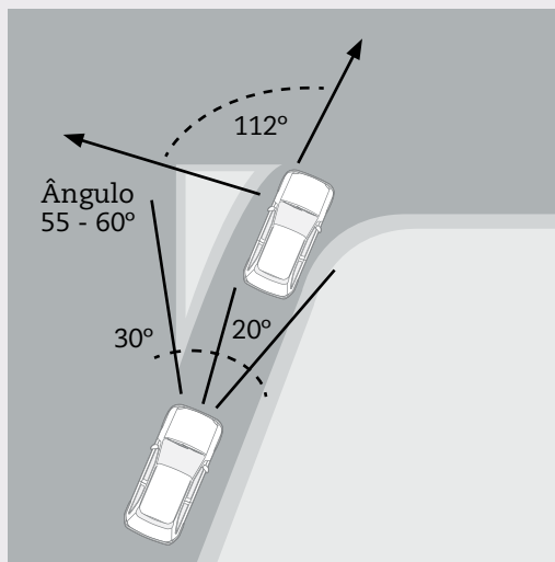
Ângulo adequado para conversão à direita. Fonte: ITDP Brasil (adaptação de FHWA, 2004 e do manual “Ciclociudades: Manual integral de movilidad ciclista para ciudades mexicanas”, publicado em 2011 pelo ITDP México).
