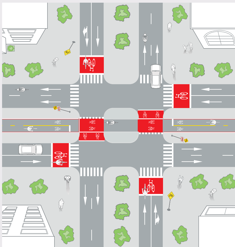
Desenho esquemático de interseção não semaforizada em ciclovia bidirecional no canteiro central, com caixas de acumulação ocupando duas faixas de rolamento em sentido único para permitir conversões de ciclistas à direita e à esquerda. Fonte: ITDP Brasil (adaptação do manual “Ciclociudades: Manual integral de movilidad ciclista para ciudades mexicanas”, publicado em 2011 pelo ITDP México).
