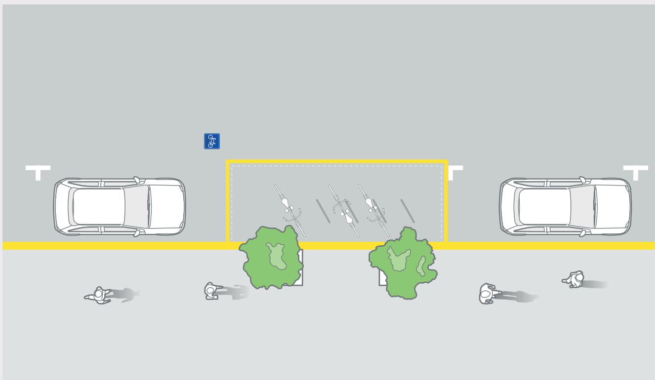
Desenho esquemático de paraciclos instalados em uma vaga destinada a automóveis, em um ângulo de 60 graus em relação ao meio fio, sendo complementados com elementos balizadores e uma linha delimitadora da vaga. Fonte: ITDP Brasil (adaptação para o português das imagens originais em espanhol do manual “ Ciclociudades: Manual integral de movilidad ciclista para ciudades mexicanas ”, publicado em 2011 pelo ITDP México).
