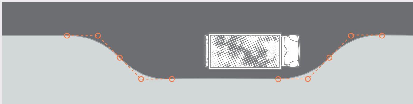
Desenho esquemático da baia para carga e descarga. Fonte: ITDP Brasil (adaptação do manual “ Ciclociudades: Manual integral de movilidad ciclista para ciudades mexicanas ”, publicado em 2011 pelo ITDP México).
