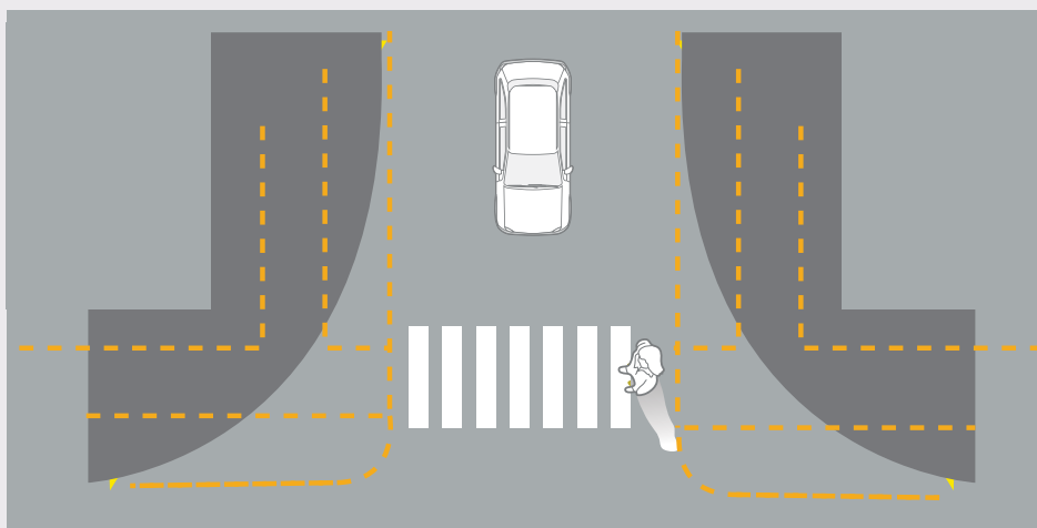
Desenho esquemático da redução dos raios de giro em interseções. Fonte: ITDP Brasil (adaptação do manual “Ciclociudades: Manual integral de movilidad ciclista para ciudades mexicanas”, publicado em 2011 pelo ITDP México).
