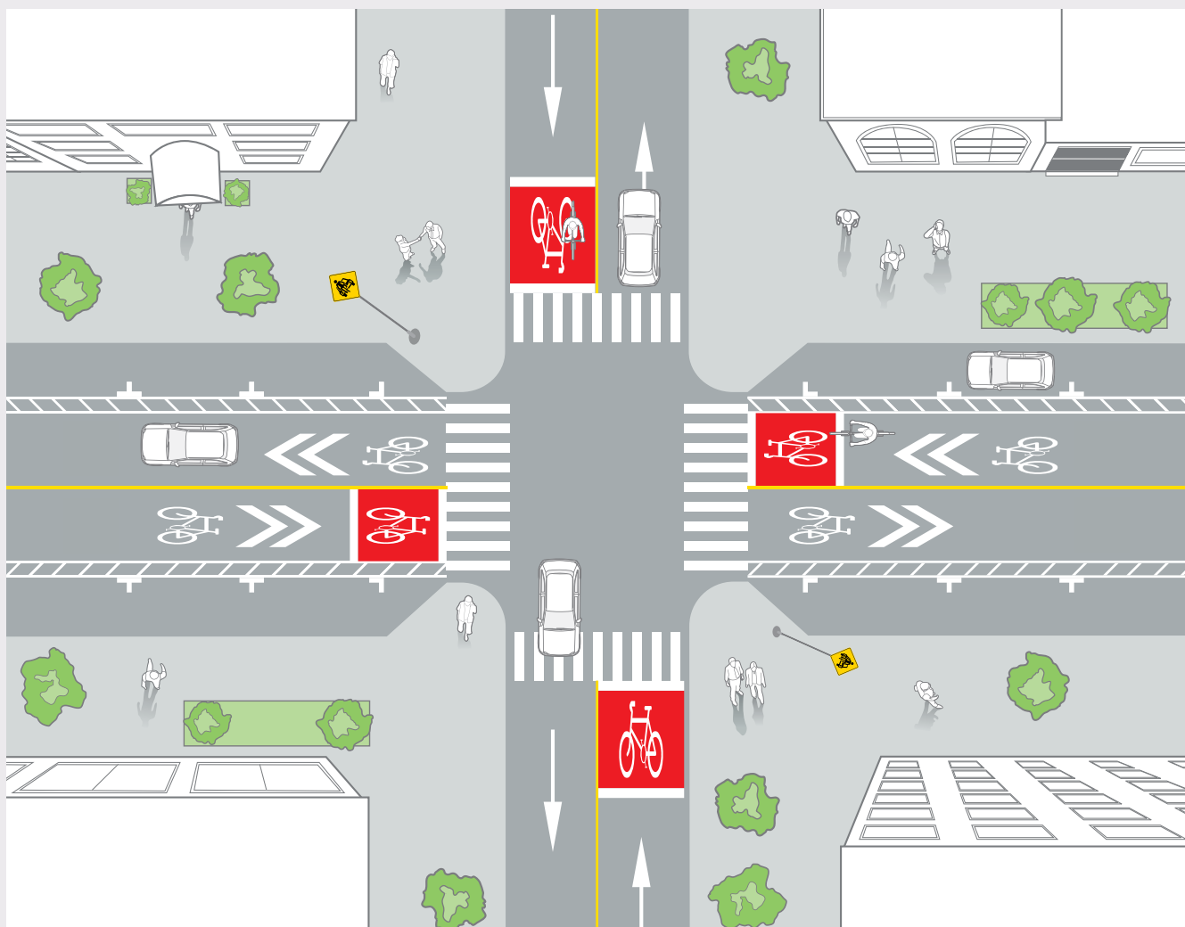
Desenho esquemático de interseção em via compartilhada. Fonte: ITDP Brasil (adaptação do manual “ Ciclociudades: Manual integral de movilidad ciclista para ciudades mexicanas ”, publicado em 2011 pelo ITDP México).
