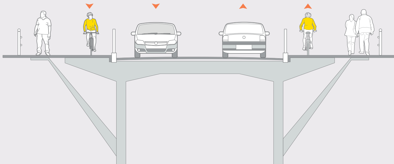
Desenho esquemático da ampliação de uma ponte destinada ao tráfego de veículos motorizados para o tráfego de pedestres e bicicletas. Fonte: ITDP Brasil (adaptação do manual “ Ciclociudades: Manual integral de movilidad ciclista para ciudades mexicanas ”, publicado em 2011 pelo ITDP México).
