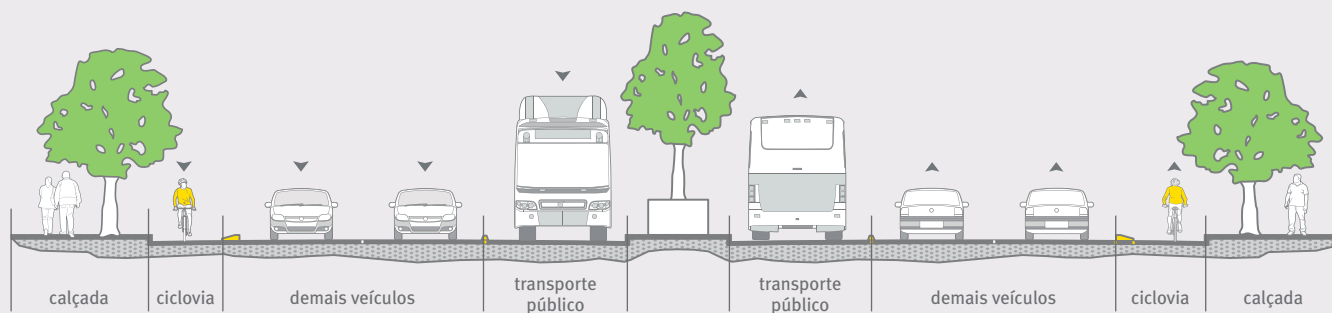
Perfil de uma via com um corredor de BRT e ciclovias unidirecionais em cada sentido. Fonte: ITDP Brasil (adaptação do manual “ Ciclociudades: Manual integral de movilidad ciclista para ciudades mexicanas ”, publicado em 2011 pelo ITDP México).
