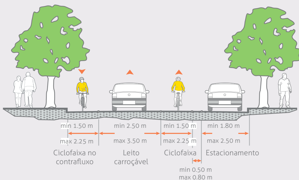
Seção de uma via unidirecional com ciclofaixas em ambos os sentidos. Fonte: ITDP Brasil (adaptação de SANZ, 1999).
