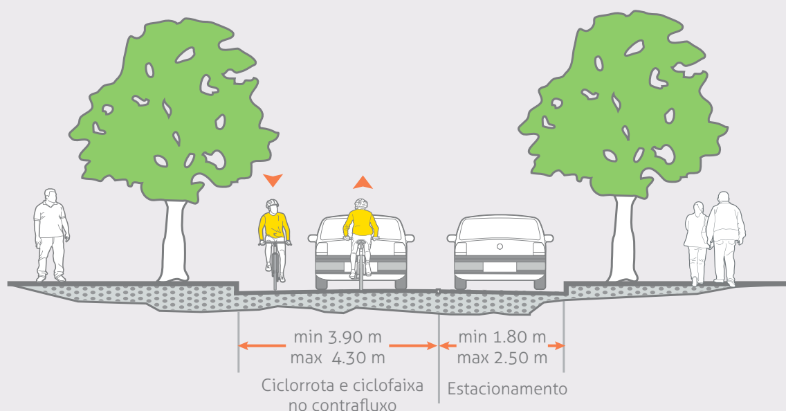
Seção de uma via unidirecional com ciclorrota e ciclofaixa no contrafluxo. Fonte: ITDP Brasil (adaptação de SANZ, 1999).
